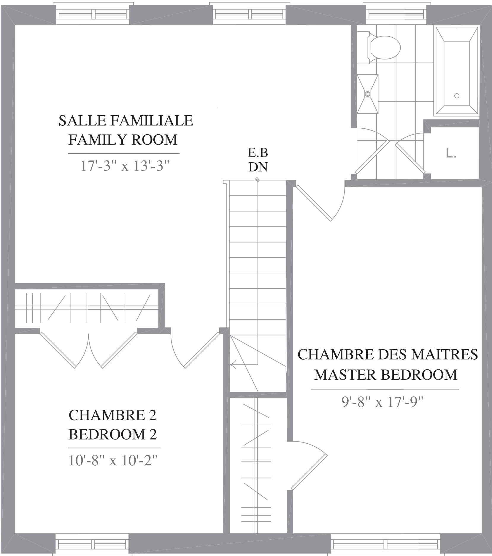
PLAN DE L'ETAGE UPPER FLOOR PLAN
