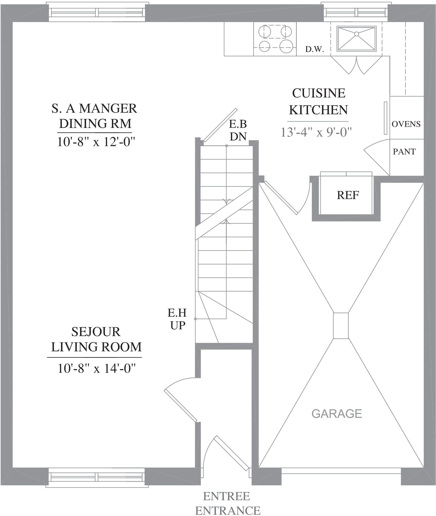
PLAN DU REZ-DE-CHAUSSEE GROUND FLOOR PLAN
