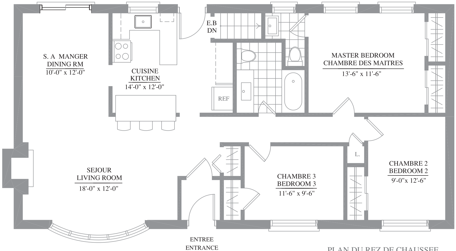
PLAN DU REZ DE CHAUSSEE MAIN FLOOR PLAN
