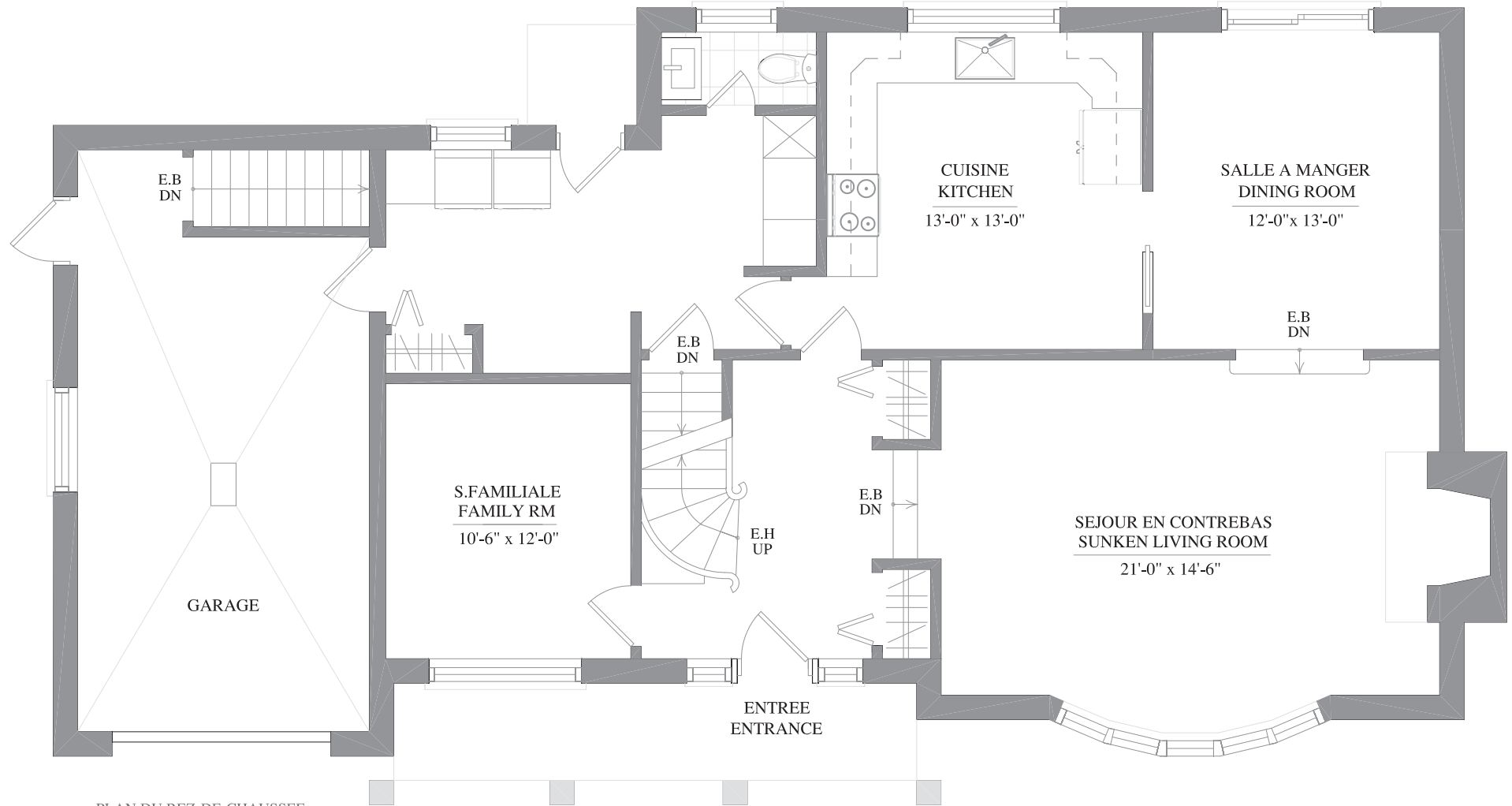
PLAN DU REZ-DE-CHAUSSEE MAIN FLOOR PLAN
