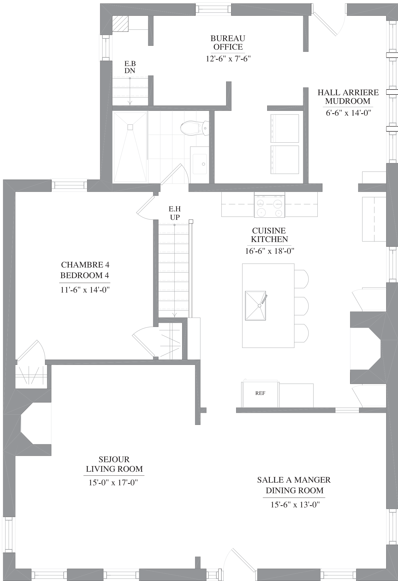
PLAN DU REZ-DE-CHAUSSEE MAIN FLOOR PLAN
