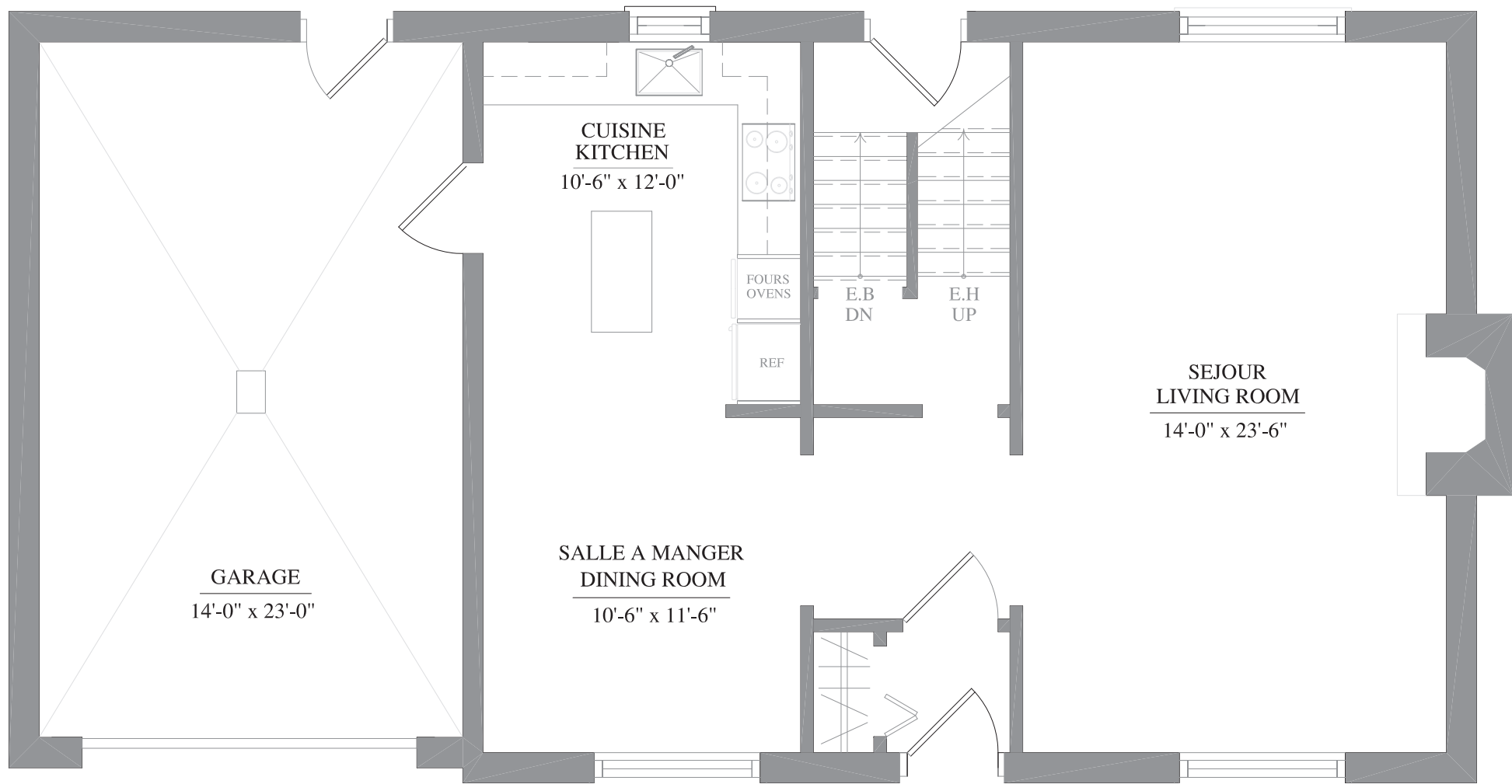
PLAN DU REZ-DE-CHAUSSEE MAIN FLOOR PLAN
