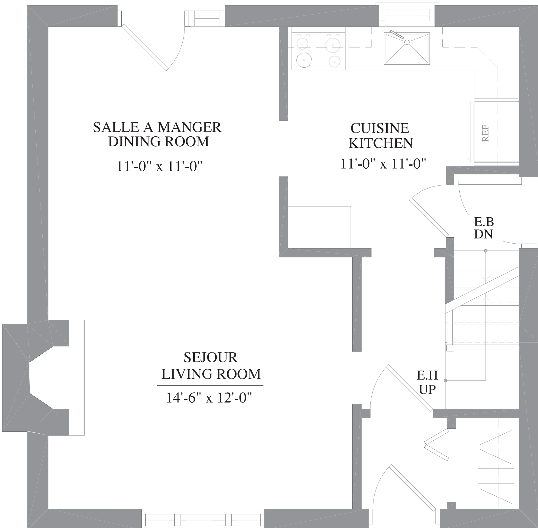
PLAN DU REZ-DE-CHAUSSEE MAIN FLOOR PLAN
