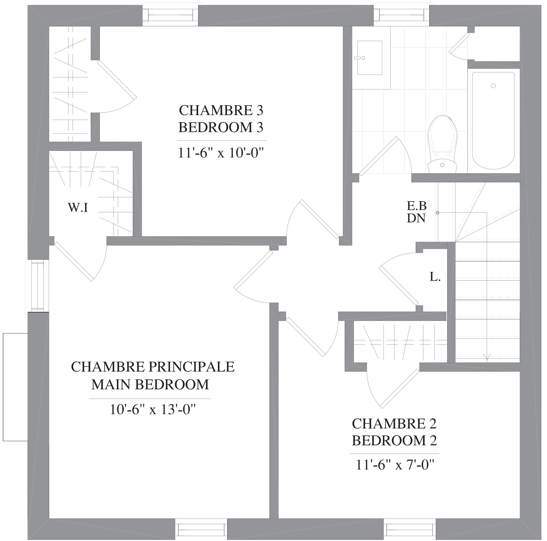
PLAN DE L'ETAGE UPPER FLOOR PLAN
