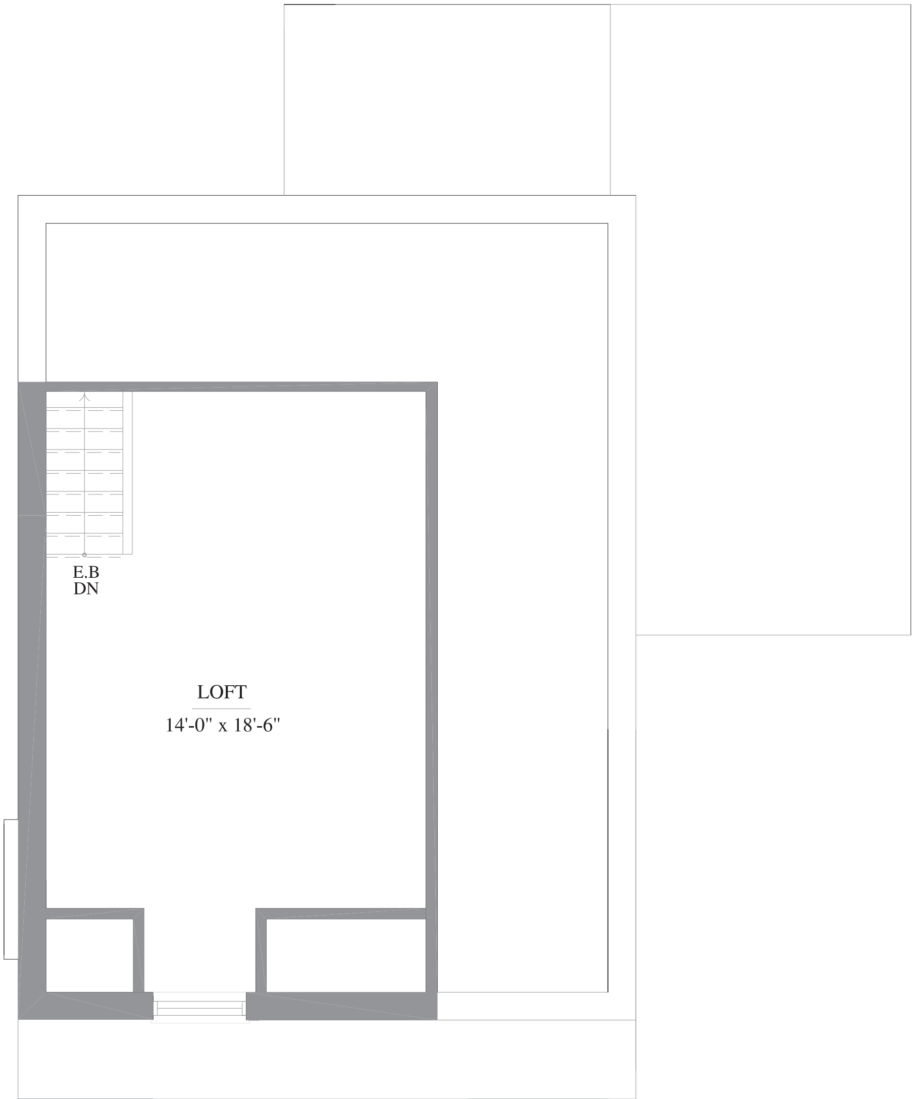
PLAN DU LOFT LOFT FLOOR PLAN
