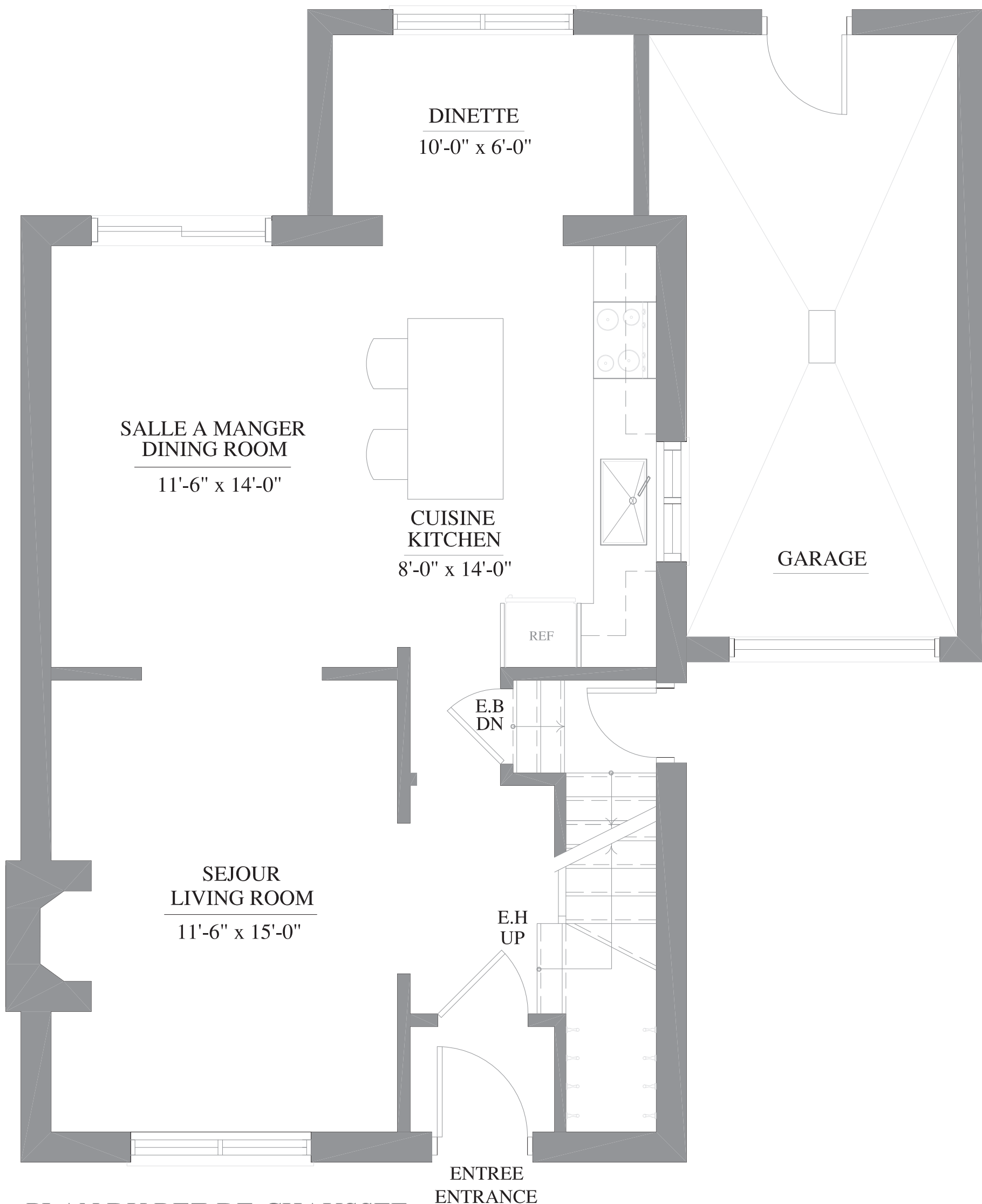
PLAN DU REZ-DE-CHAUSSEE MAIN FLOOR PLAN
