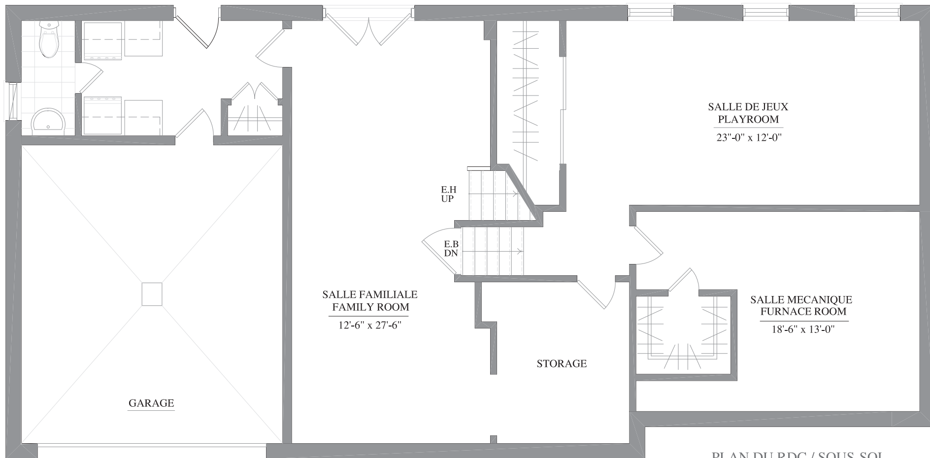
PLAN DU RDC / SOUS-SOL MAIN/LOWER FLOOR PLAN
