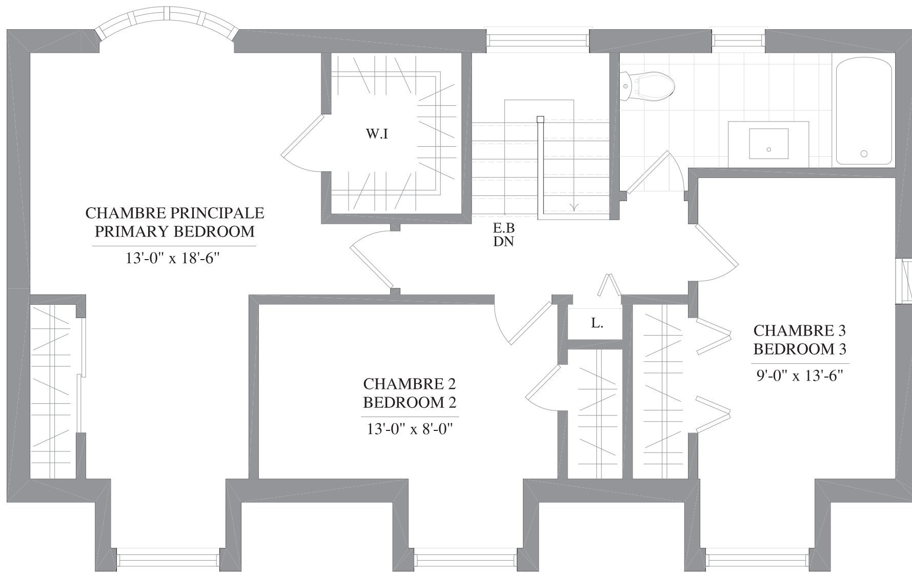
PLAN DE L'ETAGE UPPER FLOOR PLAN
