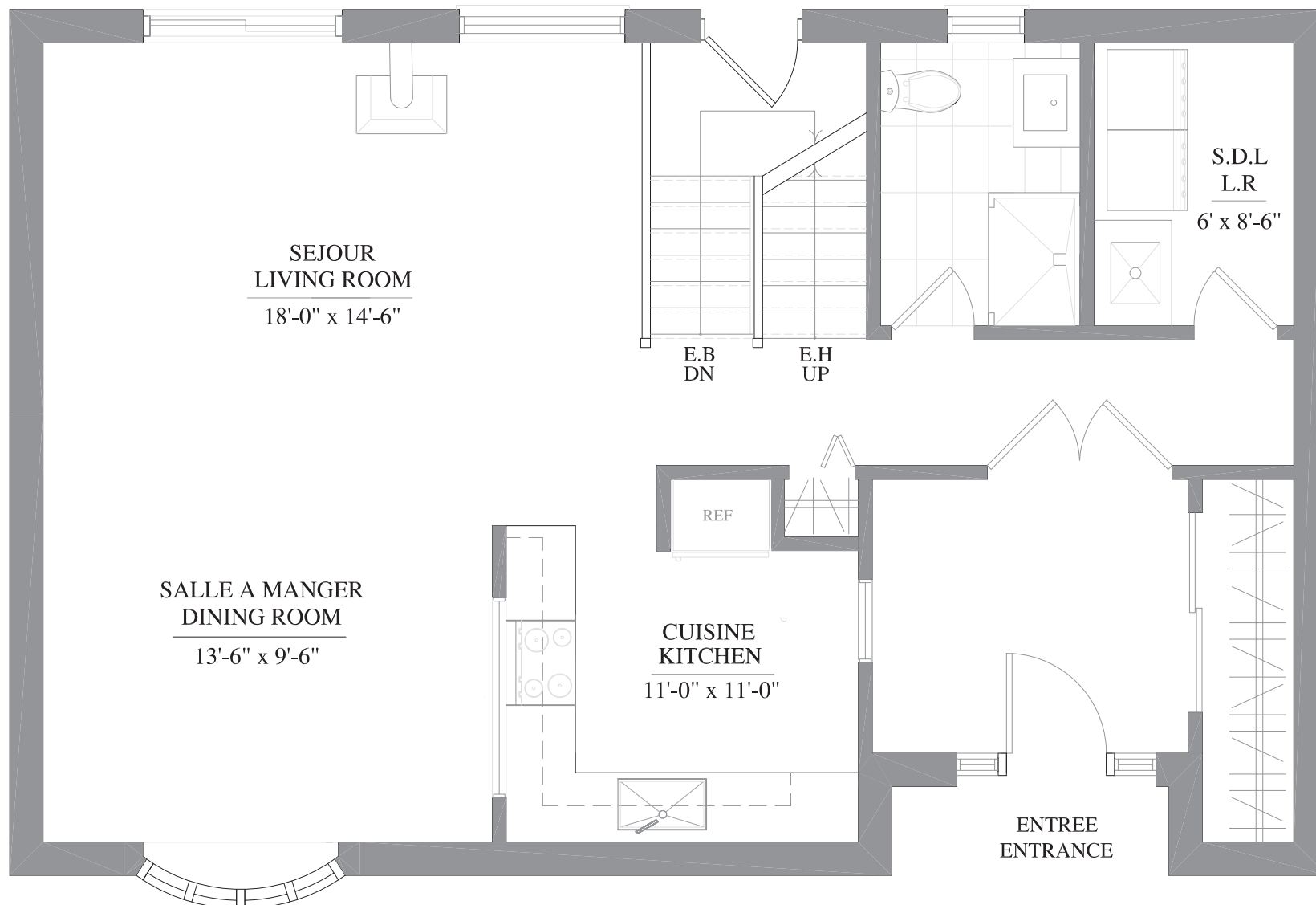
PLAN DU REZ-DE-CHAUSSEE MAIN FLOOR PLAN
