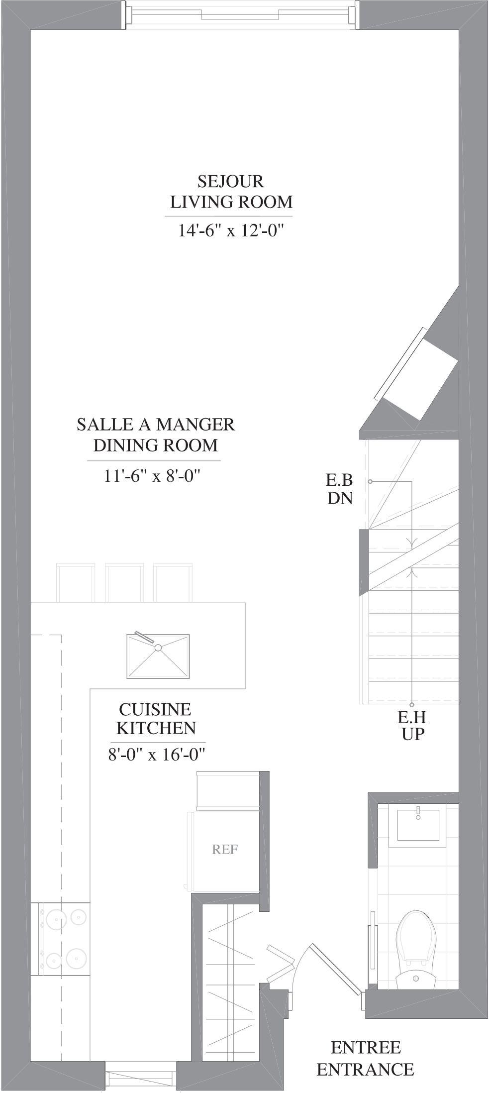
PLAN DU REZ-DE-CHAUSSEE MAIN FLOOR PLAN
