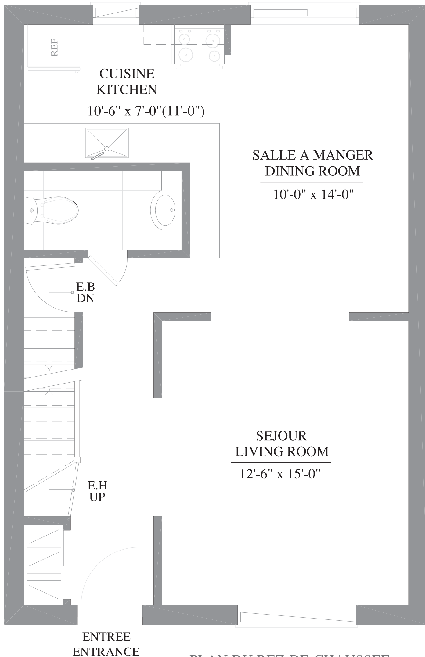
PLAN DU REZ-DE-CHAUSSEE MAIN FLOOR PLAN
