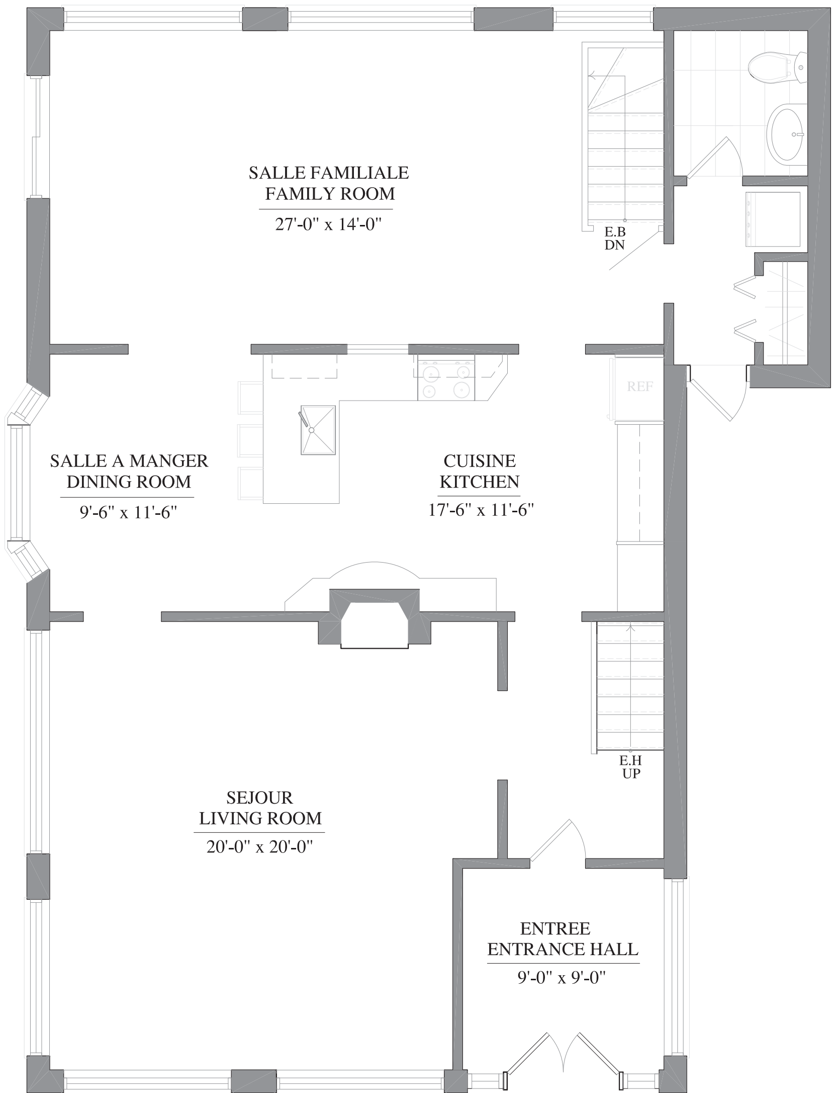
PLAN DU REZ-DE-CHAUSSEE MAIN FLOOR PLAN
