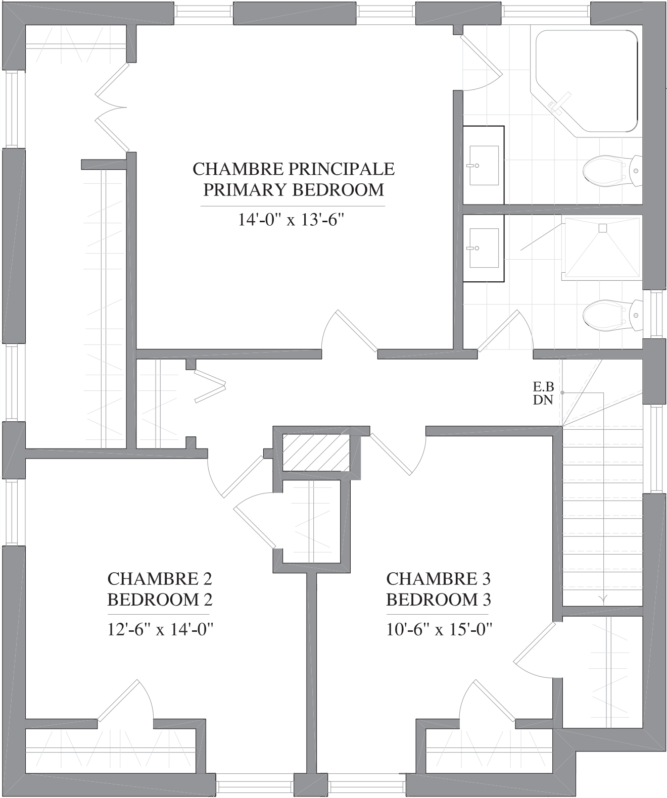
PLAN DE L'ETAGE UPPER FLOOR PLAN
