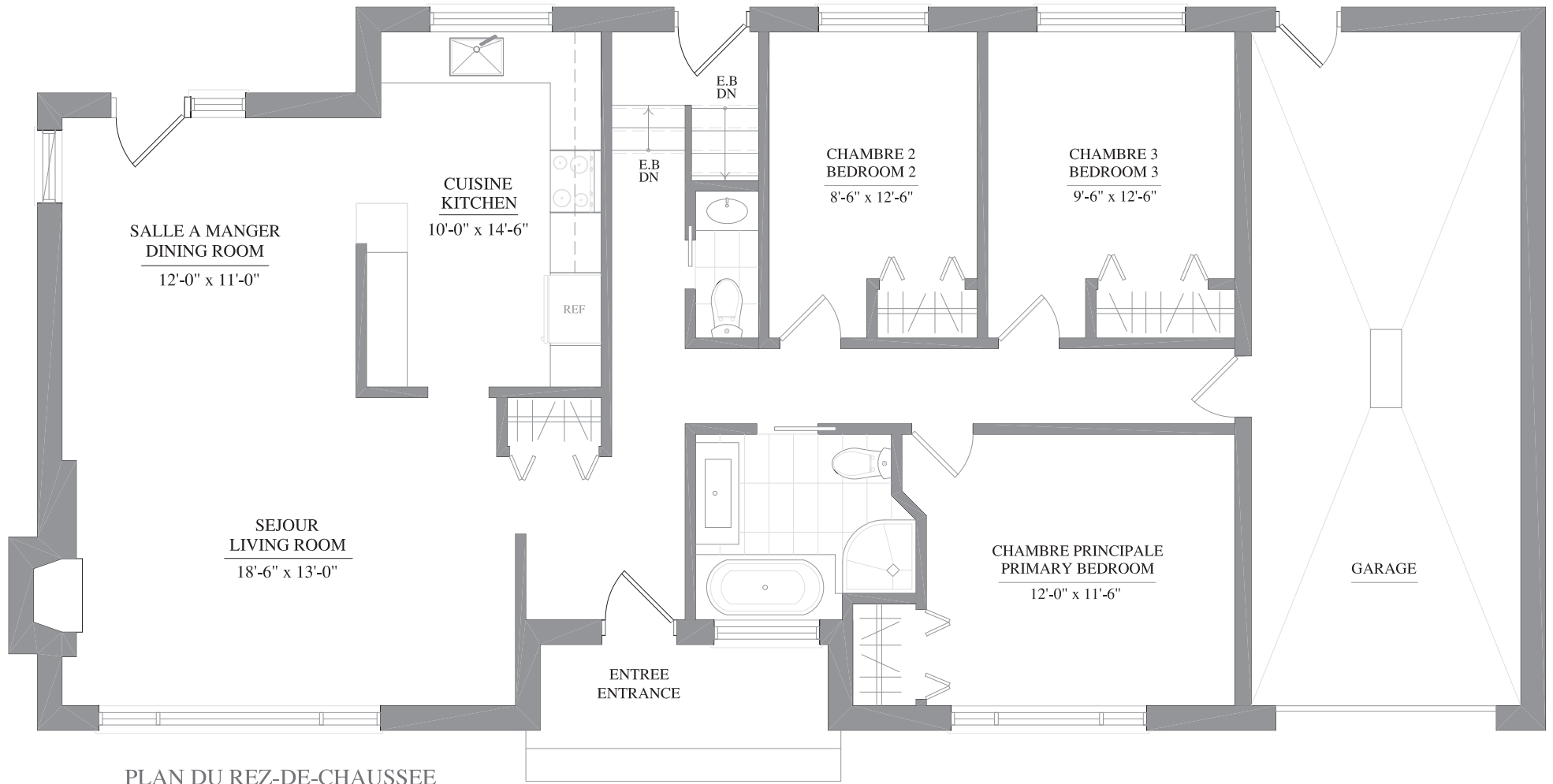
PLAN DU REZ-DE-CHAUSSEE MAIN FLOOR PLAN
