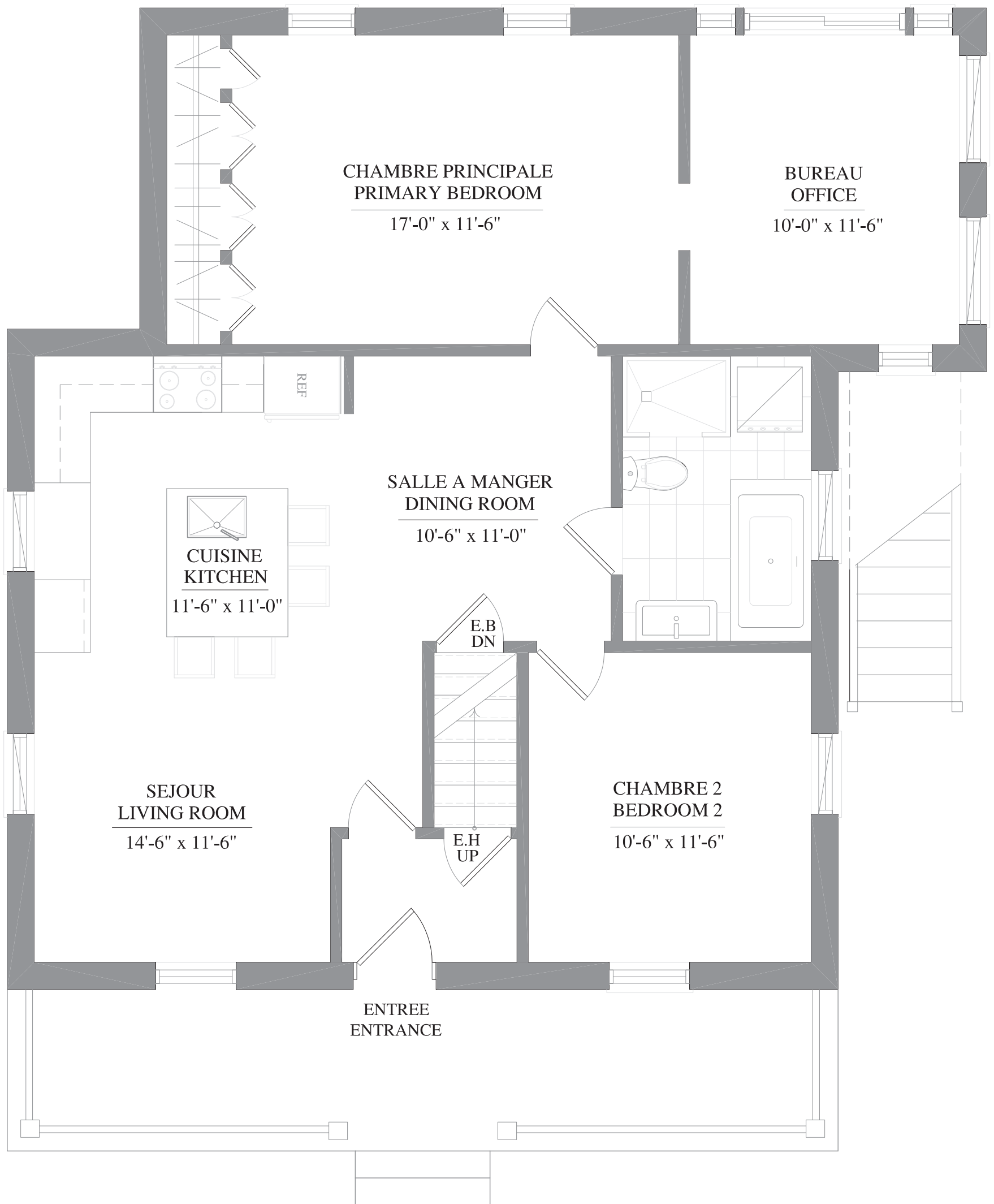
PLAN DU REZ-DE-CHAUSSEE MAIN FLOOR PLAN
