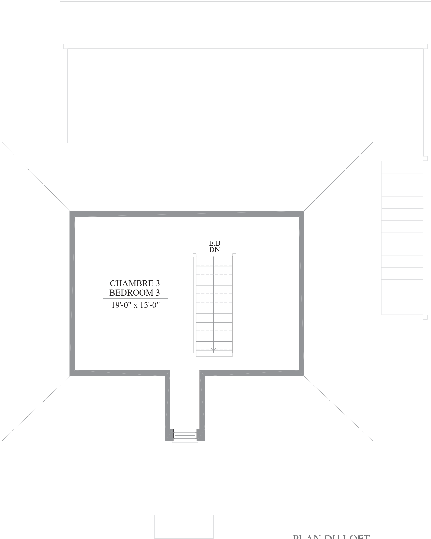
PLAN DU LOFT LOFT FLOOR PLAN
