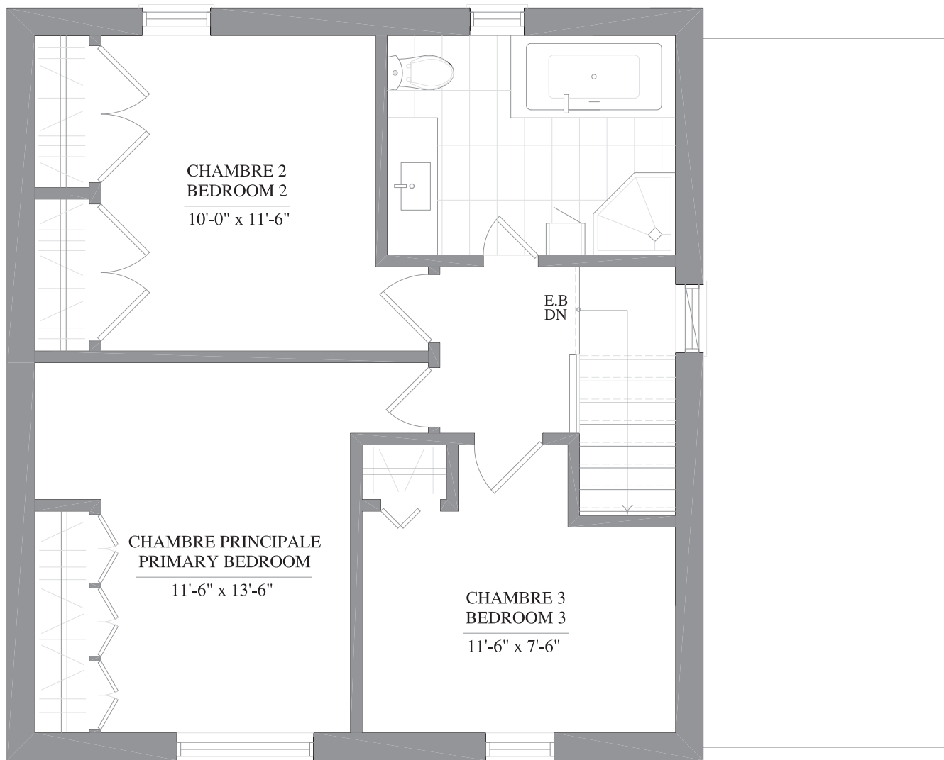
PLAN DE L'ETAGE SECOND FLOOR PLAN
